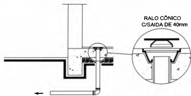
INSTALAÇÃO - RALO SIFONADO Esc 1 : 20
