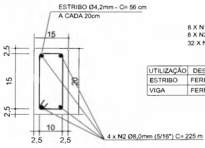
CORTE AA
