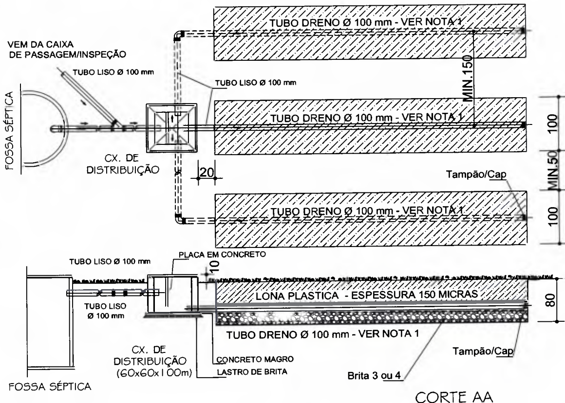
CORTE AA
