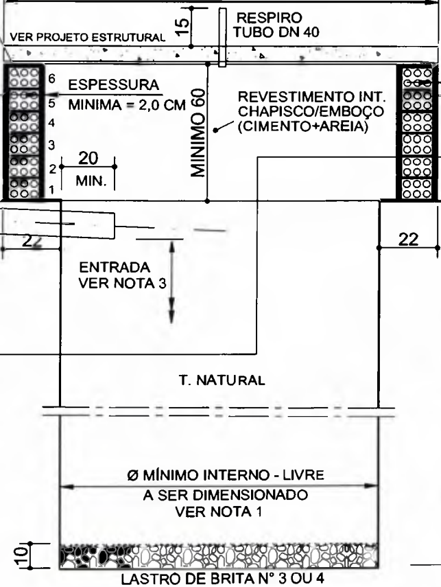
CORTE Esc 1 : 20
