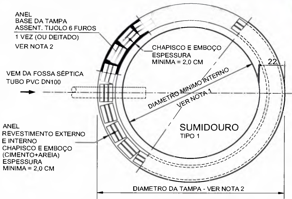
PLANTA Esc 1 : 20
