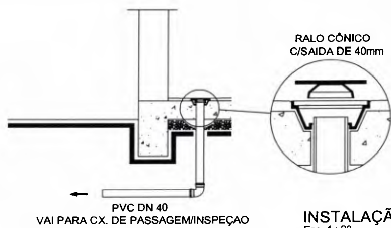
INSTALAÇÃO - CAIXA DE DESCARGA E VASO SANITÁRIO Esc 1 : 20
