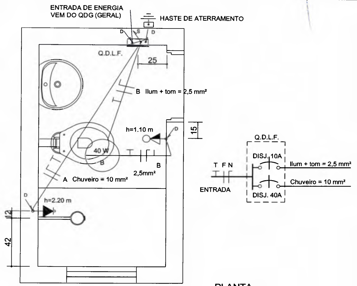
PLANTA Esc 1 : 20
